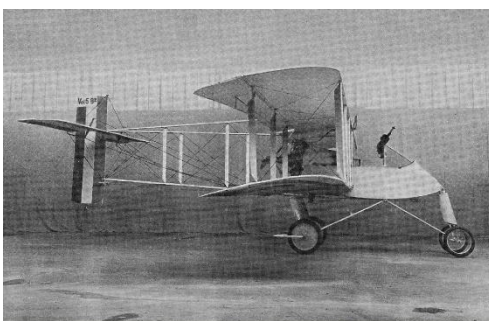
J'ai piloté ce Voisin à la V.B. 107 le 1er sept. 1915 jusqu'en mai 1917. Bombardements de jour à l'abord et de nuit ensuite. Incroyable mécanique avec son moteur Bantou 1100 cc de 130 ch.
